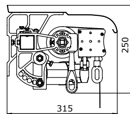
Kotvenie na čelnú stenu so strieškou
