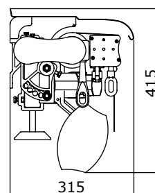
Kotvenie na čelnú stenu so strieškou
