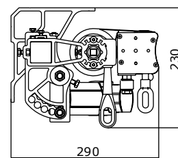
Stropné kotvenie
