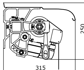
Kotvenie na čelnú stenu so strieškou
