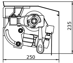
Kotvenie na čelnú stenu so strieškou
