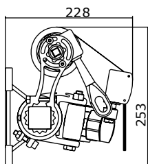
Kotvenie na čelnú stenu
