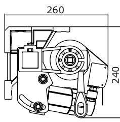
Kotvenie do stropu
