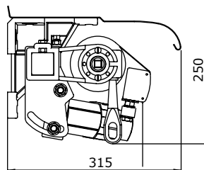
Kotvenie na čelnú stenu so strieškou
