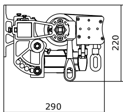
Kotvenie na čelnú stenu
