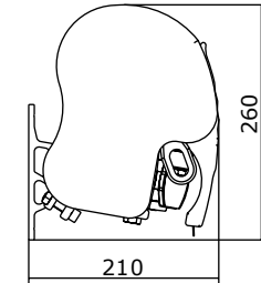
Kotvenie na čelnú stenu
